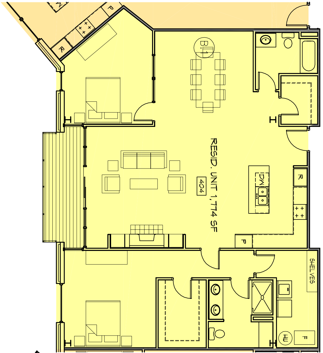
4 LIVING UNITS 404 SCALE: 1/8"=1'-0"
