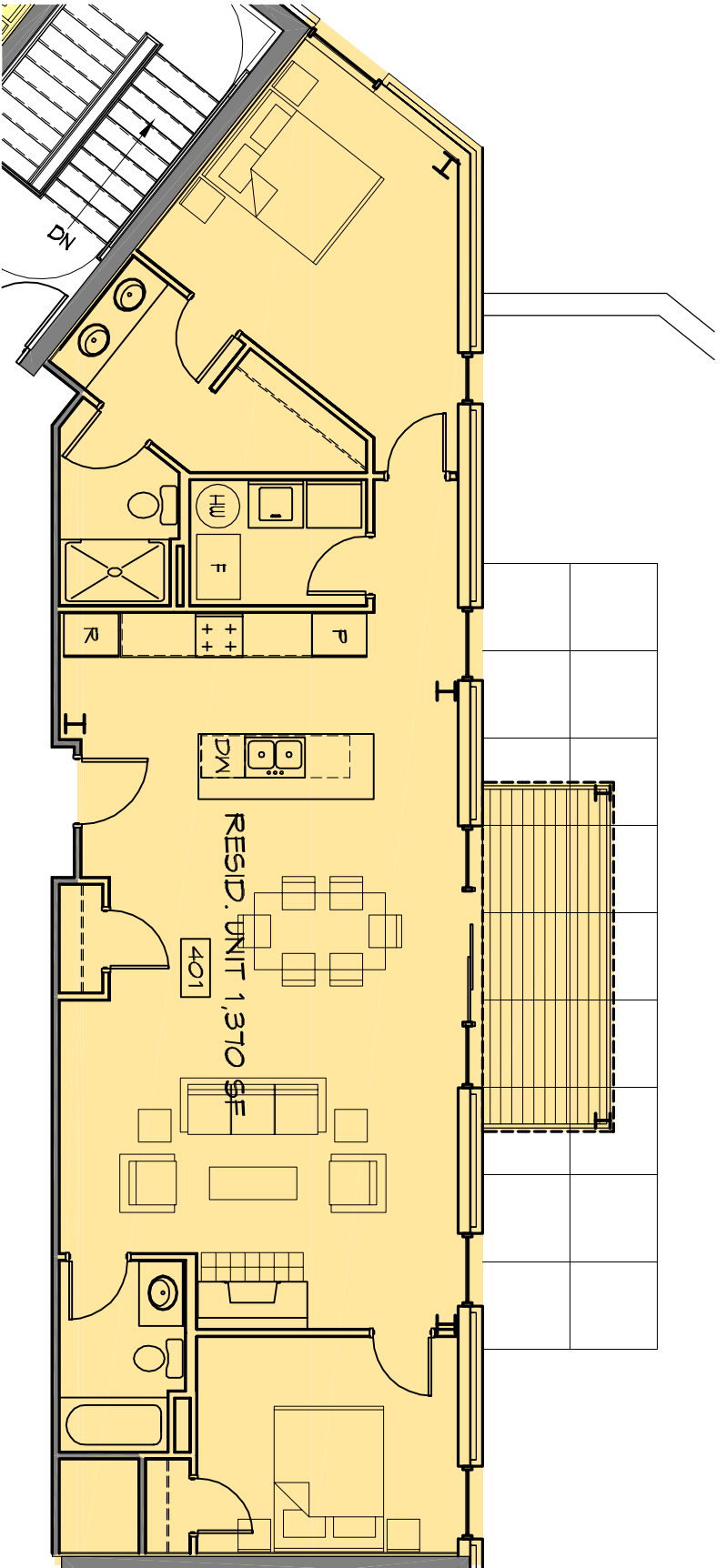
1 LIVING UNIT 401 SCALE: 1/8"=1'-0"
