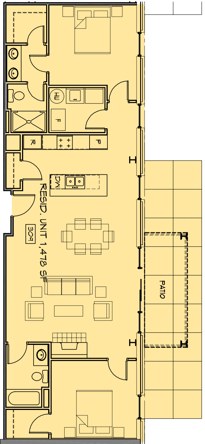
9 LIVING UNIT 309 SCALE: 1/8"=1'-0"
